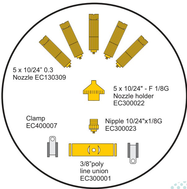
MOST COMMON PARTS FOR FOG EFFECTS ПРИМЕР КОМПЛЕКТАЦИИ ДЛЯ ЭФФЕКТА ТУМАНА
