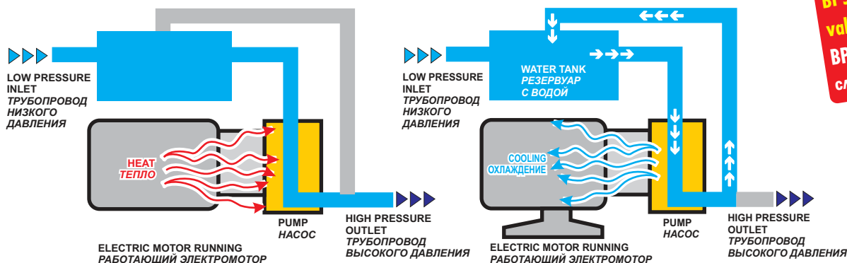
BPS WORKING PRINCIPLE - ПРИНЦИП РАБОТЫ СИСТЕМЫ BPS (Байпас)
