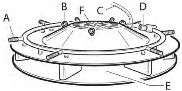
А-Форсунки-Nozzles, В=Петли для подвешивания-Chain Hooks-, С=Провод электрич.-Electric cable, D=Подвод воды-Water inlet, E=Вытяжные отверстия-Air outlet, F=Приточное отверстие-Air inlet
