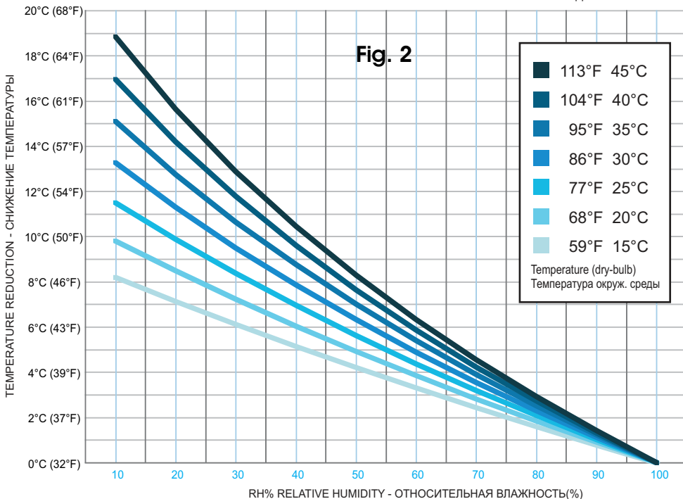
EVAPORATIVE COOLING PERFORMANCE - ПОКАЗАТЕЛИ СИСТЕМЫ ТУМАННООХЛАЖДЕНИЯ
