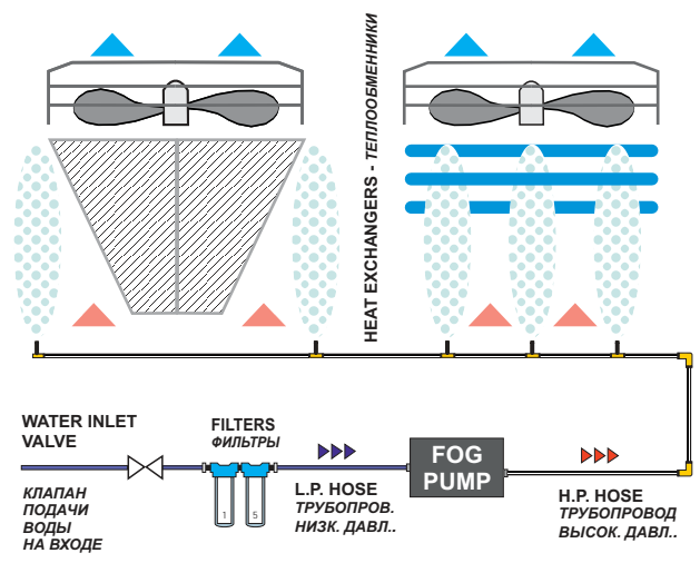
Схема монтажа предварительного охлаждения обменников Heat exchangers mounting layout example
